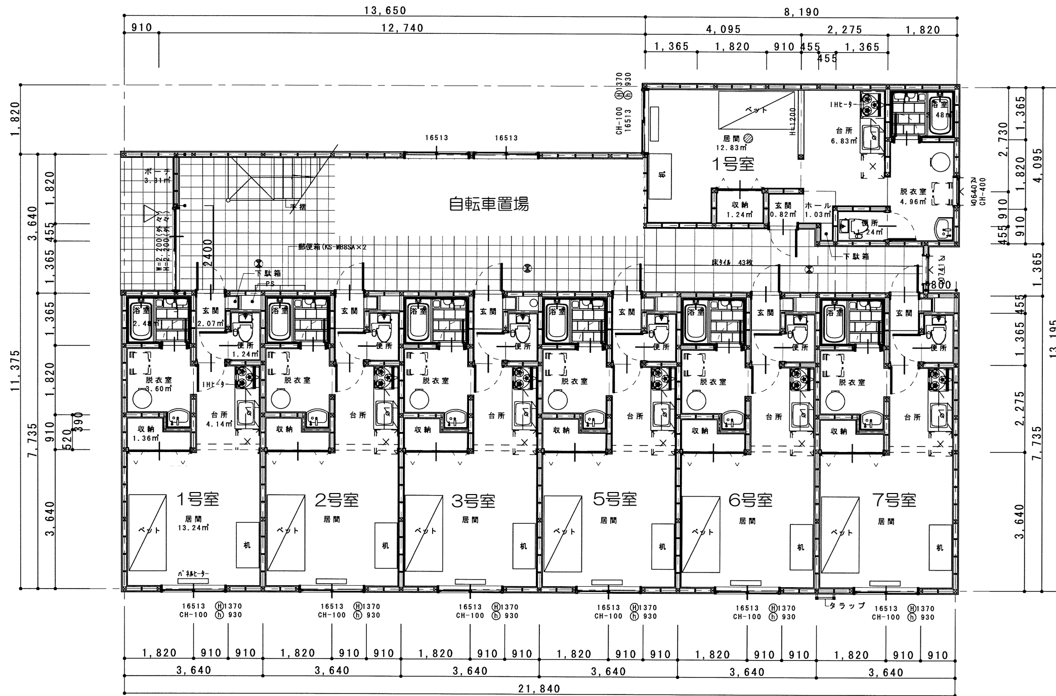
1階平面図 1/100
